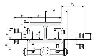
Model HTP/G 500 - 5000kg, s blokovacím zariadením
