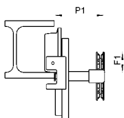
Model HTG 10000kg, blokovacie zariadenie
